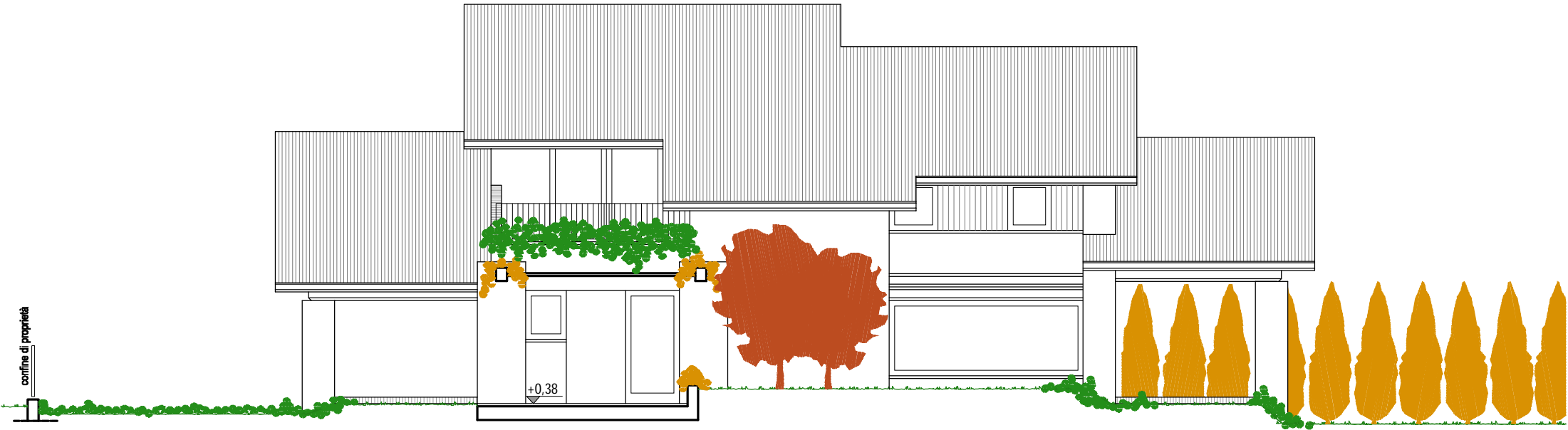
Prospetto sud-ovest rapp. 1:100
