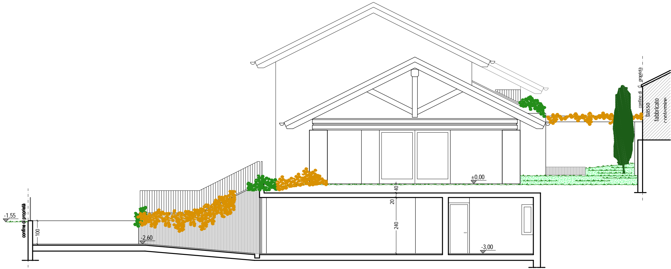
Prospetto nord-ovest rapp. 1:100
