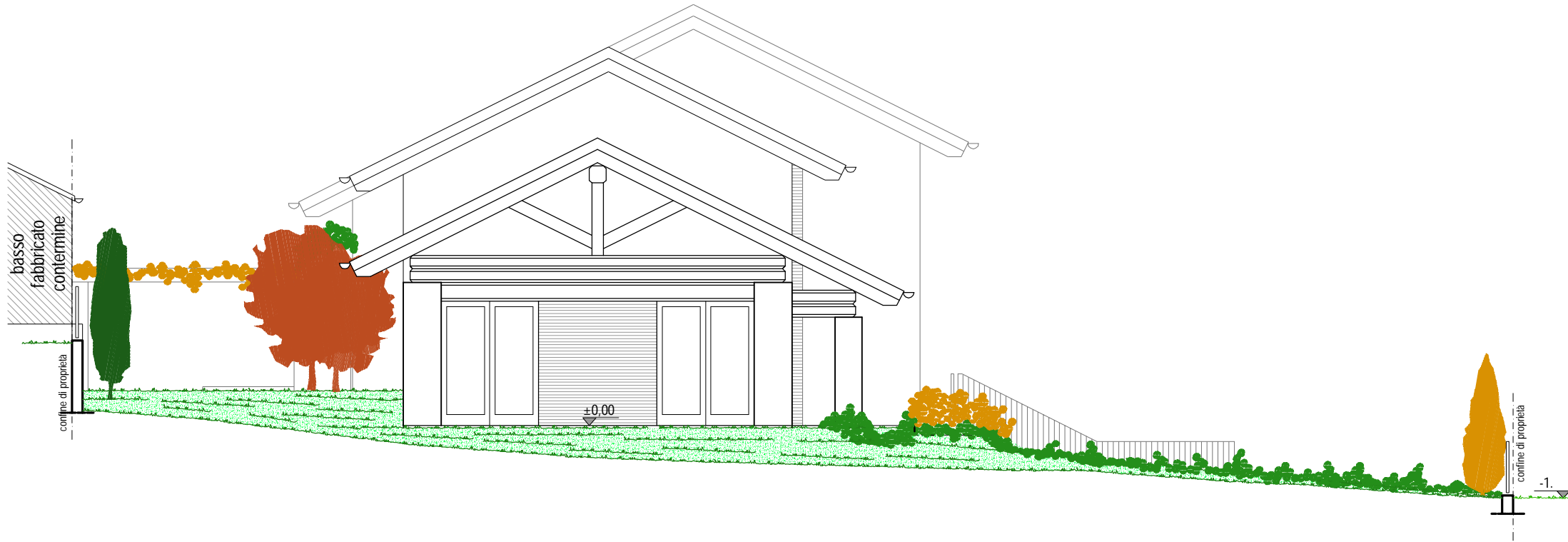
Prospetto sud-est rapp. 1:100
